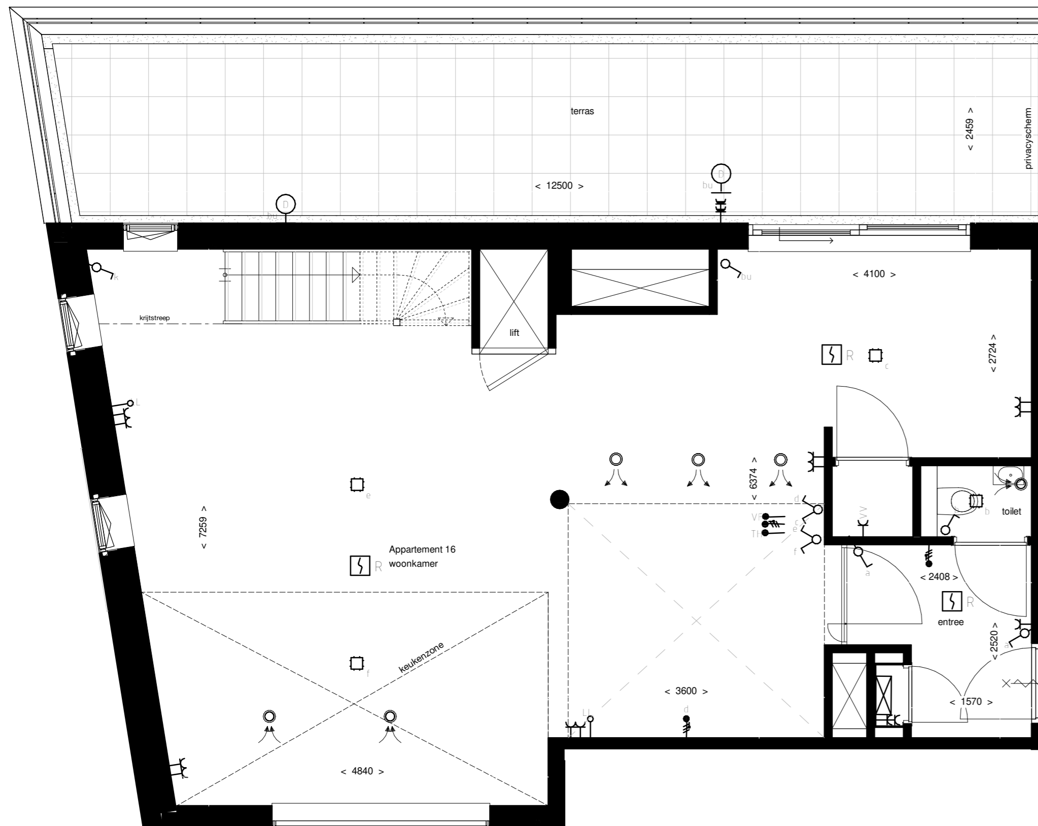
5e verdieping
