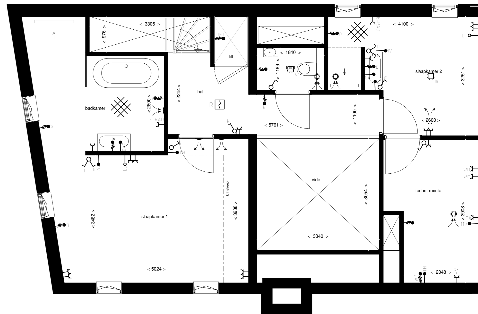
6e verdieping
